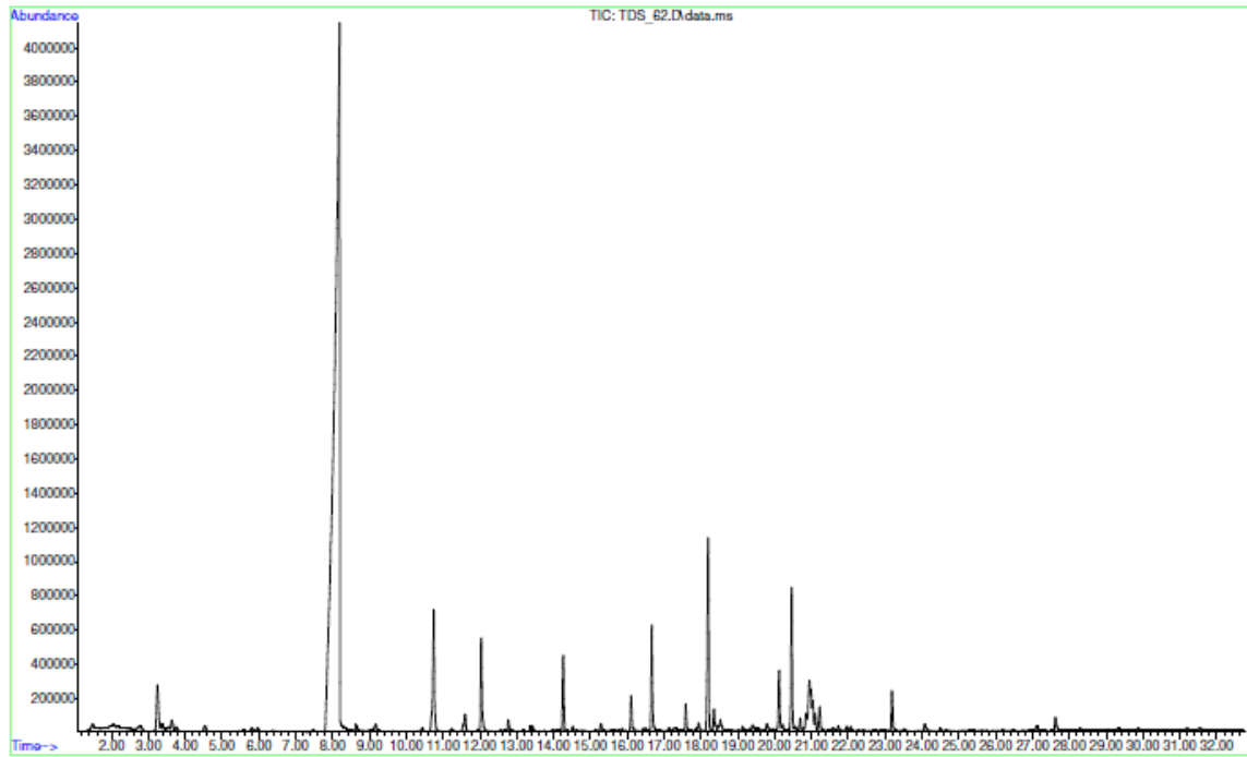
Chromatogramm
